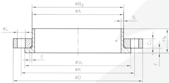
Overschuifflenzen EN1092-1/type 2 PN40
