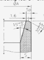
Uitvoering voor S > DN125
