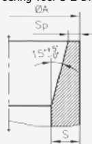
Uitvoering voor S \leq DN125
